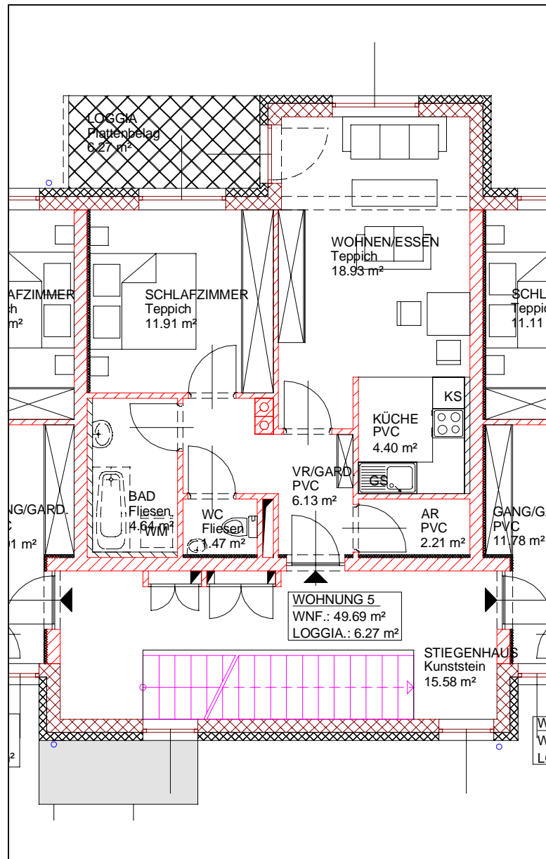
GRUNDRISS M1:100
