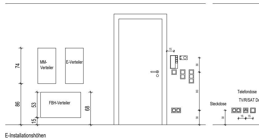
E-Installationshöhen
